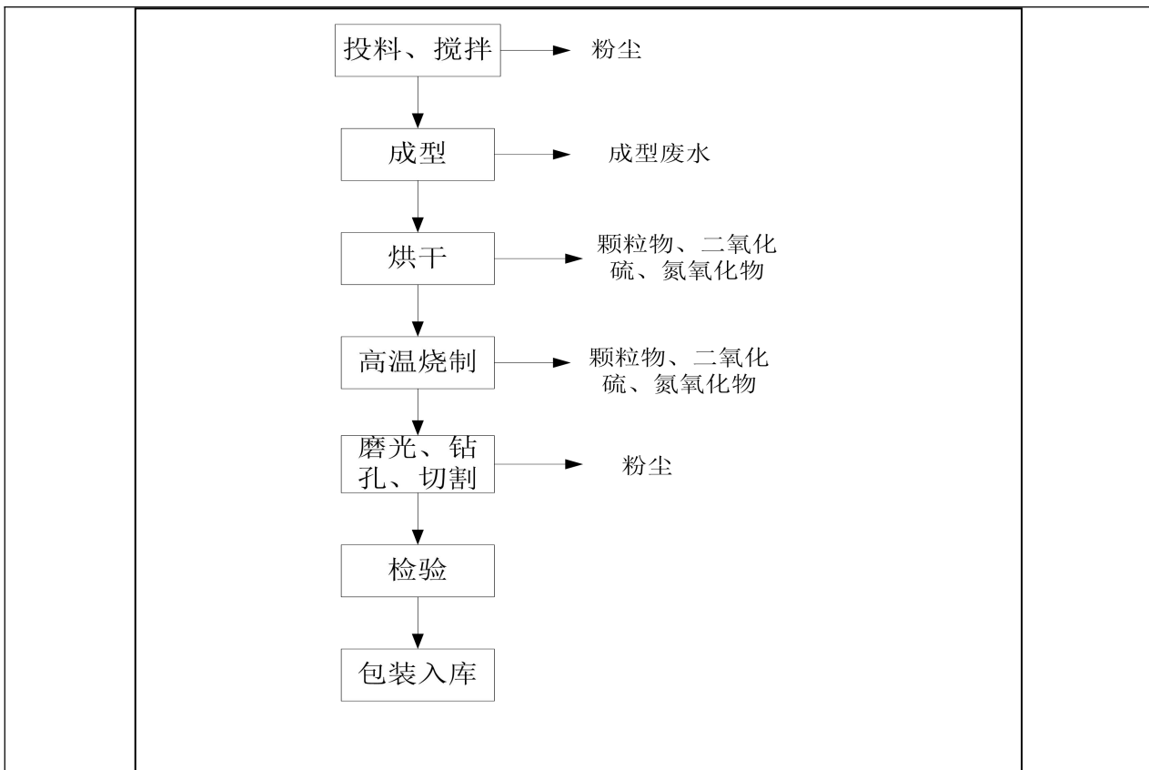
图 2-4 多晶莫来石纤维制品生产工艺流程及产污节点图
