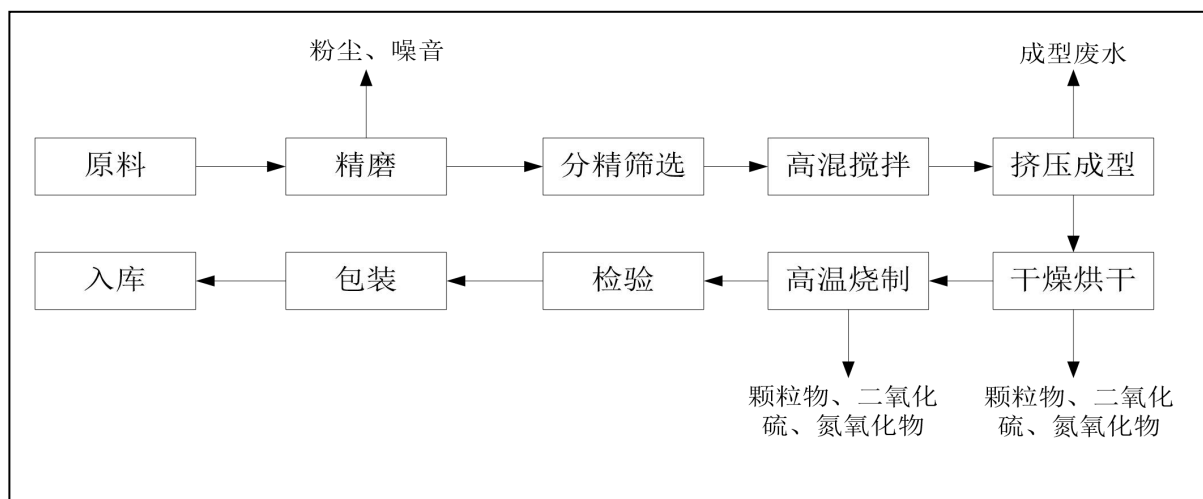
图 2-3 高端耐火材料制品生产工艺流程及产污节点图
